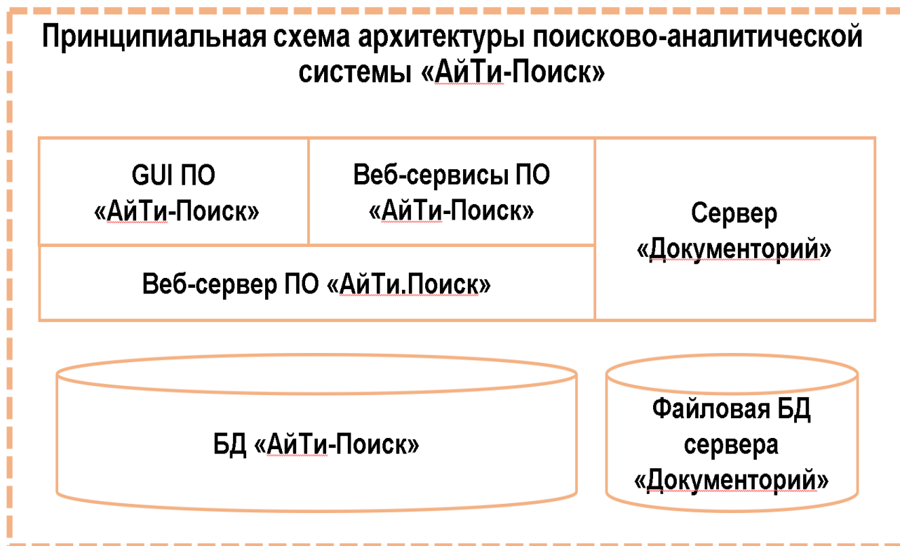
Рисунок 1. Схема концептуальной архитектуры
